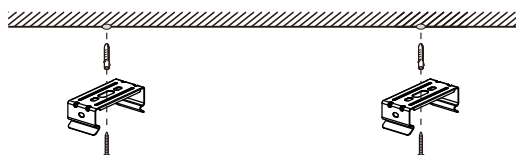
2. I henhold til senterposisjonen for monteringsfestet: Installer ekspansjonsbolter eller skruer, og monter brakettene. / According to the Fixing hole centre, instal expansion bolts and screws, instal the bracket.
