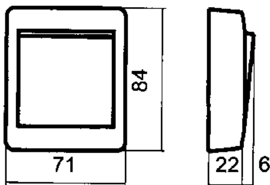
Måttitning
