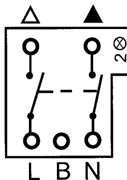
Kopplingsschema
