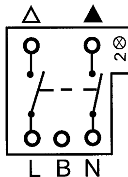
Kopplingsschema
