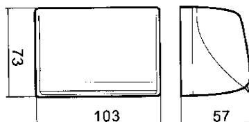
Måttritning
